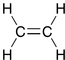
Αιθυλένιο C_2H_4
