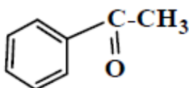
Ακετοφαινόνη
