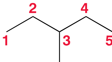
3 -Μεθυλοπεντάνιο
