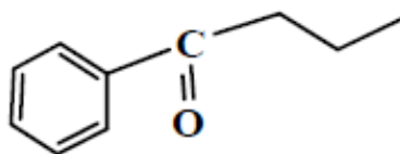
Βουτυροφαινόνη ή 1-Φαινυλο-1-βουτανόνη
