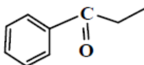
Προπιοφαινόνη
