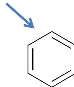
Βενζόλιο C_6H_6
