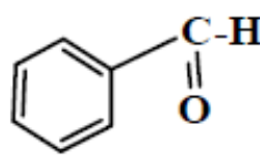
Βενζαλδεύδη
