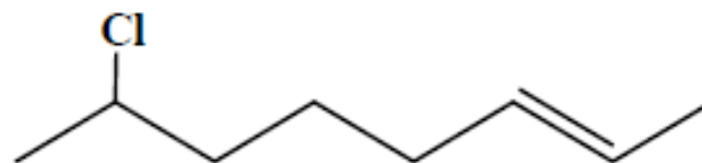
(E)-7-Χλωροοκτ-2-ένιο
