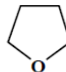
Οξολάνιο ή Τετραυδροφουράνιο
