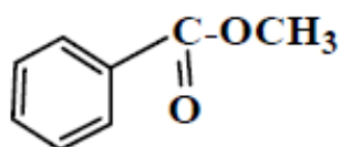
Βενζοϊκός Μεθυλεστέρας
