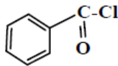
Βενζουλοχλωρίδιο
