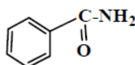
Βενζαμίδιο
