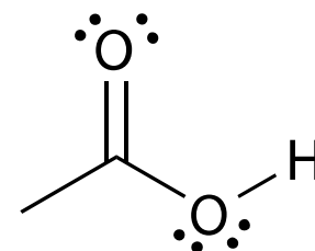
Οξικό οξύ
