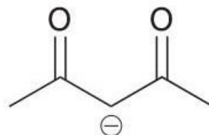
Βάση
