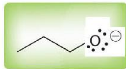
Συζυγής βάση
