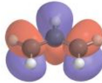
Αντι- δεσμικό MO
