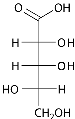
Προβολή Fischer
