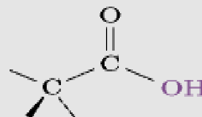
Καρβοξυλικό οξύ
