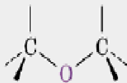
Αιθέρας
