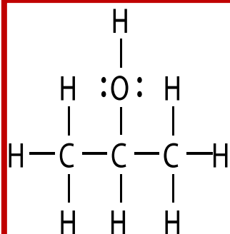
Δομή Lewis
