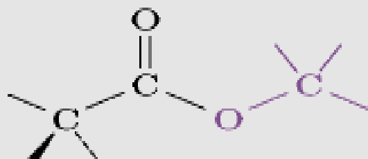
Εστέρας
