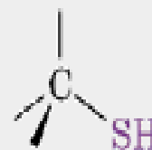
Θειόλη
