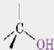
Αλκοόλη
