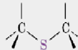
Σουλφίδιο
