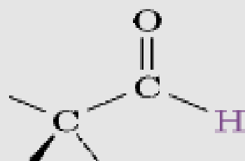
Αλδεϋδη
