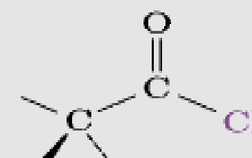
Χλωρίδιο οξέος
