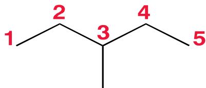
3-Μεθυλοπεντάνιο
