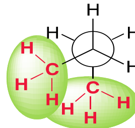
Gauche
