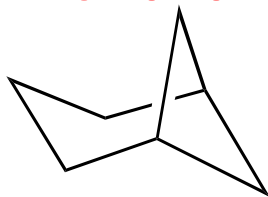
Δικυκλο[3.1.1]επτάνιο
