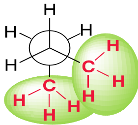
Gauche
